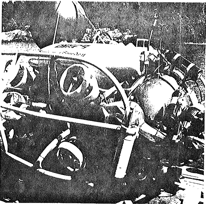
□ En självgående och enmansbetjänad dykfarkost typ Mantis, som medförs på vår nyaste minutläggare, MUL 20 Furusund. Främst används farkosten vid arbeten med fasta anordningar för undervattensbevakning och i kontrollerbara mineringar.
