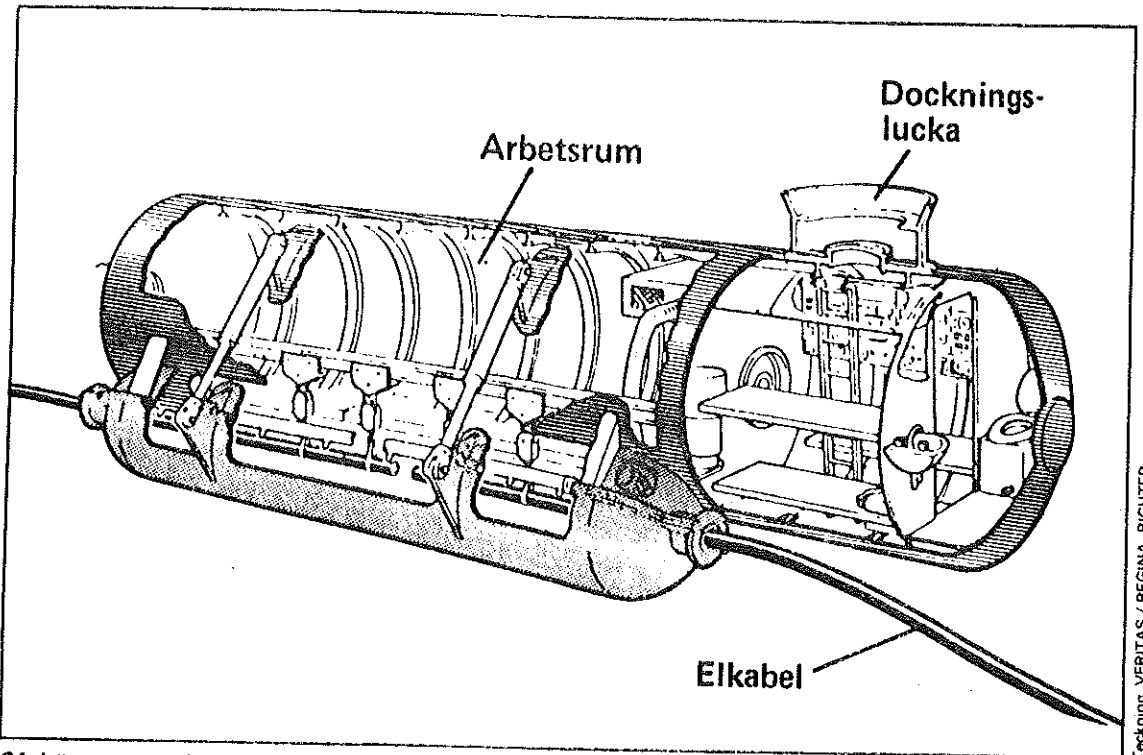
Så här ser resultatet av fransk-engelskt samarbete under vattnet ut: ett så kallat habitat, där ett gäng reparatörer ska jobba med kabelskarvning på botten av Engelska kanalen.
